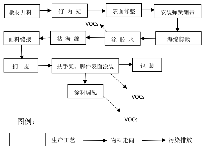
图 4-2 软体家具生产工艺流程
